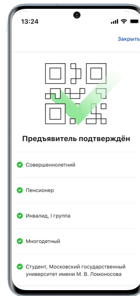
Кассовое ПО
